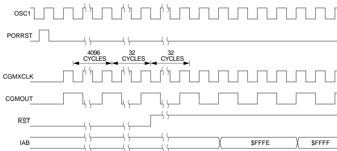
Figure 6. POR recovery
