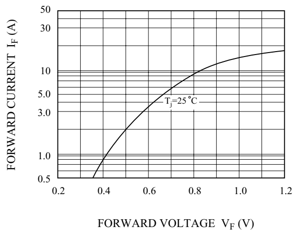
I_F - V_F
