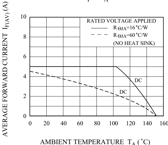
I_F - T_A
