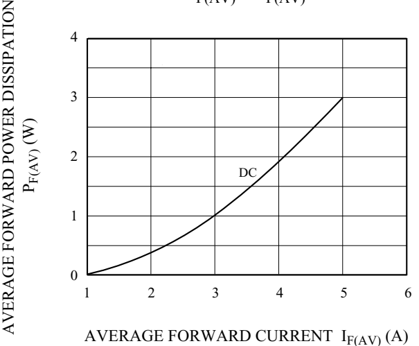
P_{F(AV)} - I_{F(AV)}
