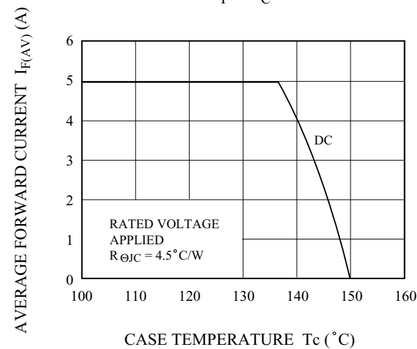
I_F - T_C
