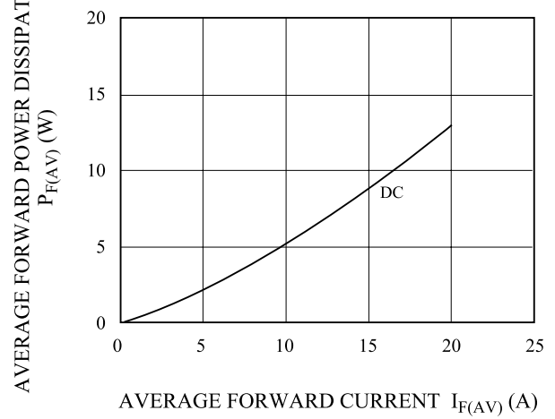
P_{F(AV)} - I_{F(AV)}
