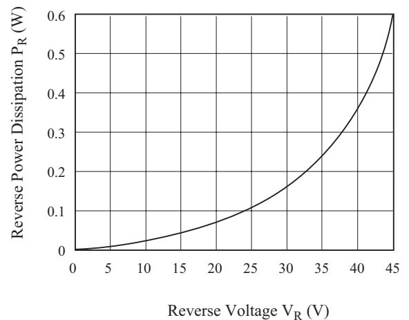
P_R - V_R
