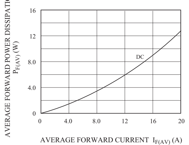
P_{F(AV)} - I_{F(AV)}
