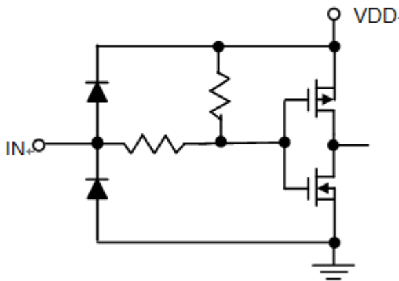
EN terminal
