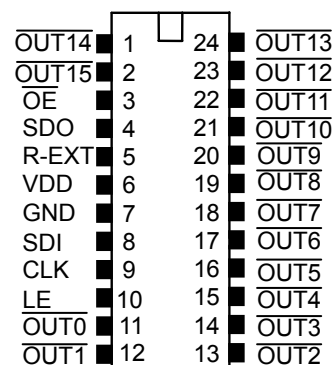
MBI5026GPA
