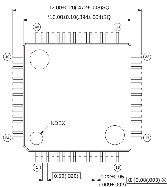
64-pin plastic LQFP (FPT-64P-M38)
