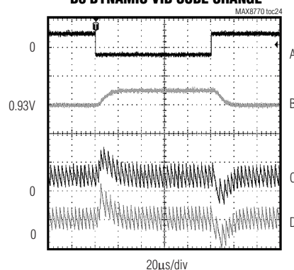
D3 DYNAMIC VID CODE CHANGE
