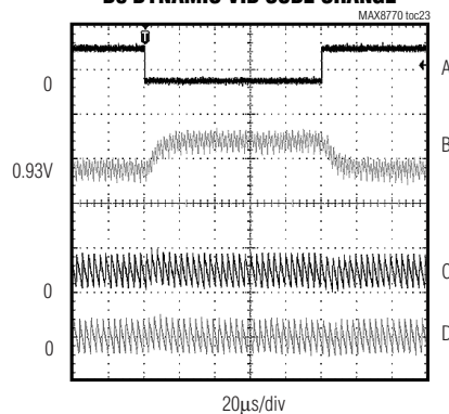
D0 DYNAMIC VID CODE CHANGE
