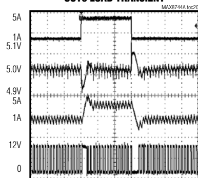
OUT5 LOAD TRANSIENT
