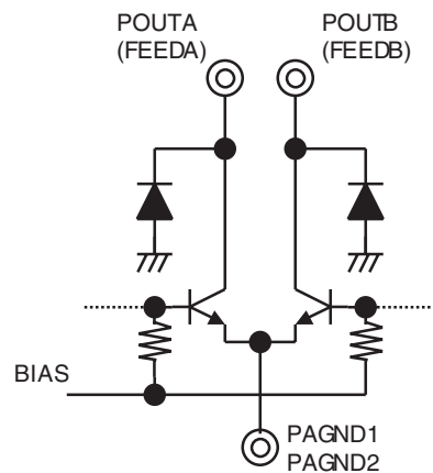
8 POUTA,POUTB,FEEDA,FEEDB
