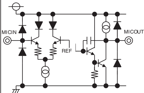
11 MICIN , MICOUT
