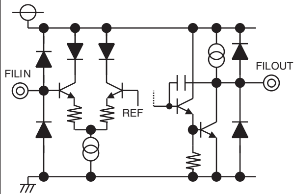
10 FILIN , FILOUT
