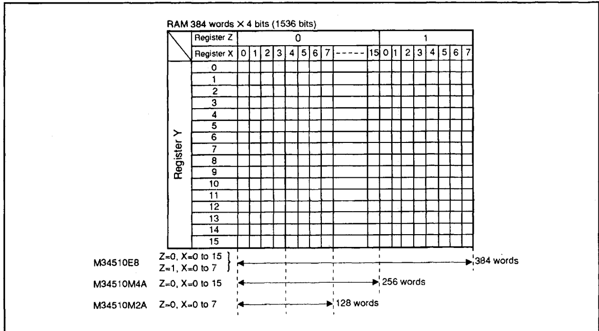
Fig. 12 RAM map
