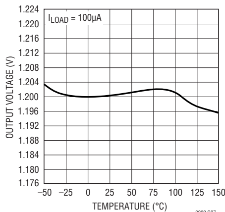
Output Voltage LT3009-1.2
