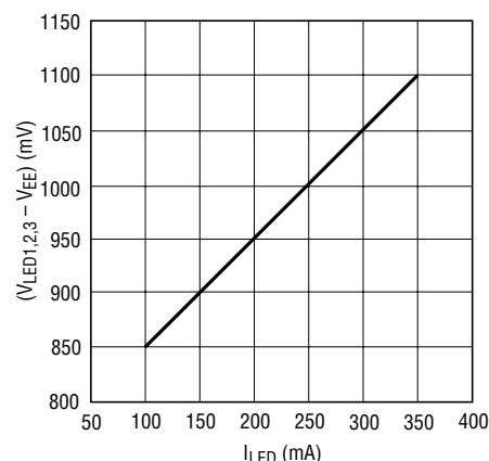
(V_{\text{LED1,2,3}} - V_{\text{EE}}) vs I_{\text{LED}}
