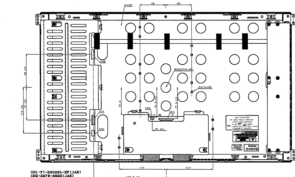
図1. LQ255T3LZ11 TFT-LCDモジュール外形図
