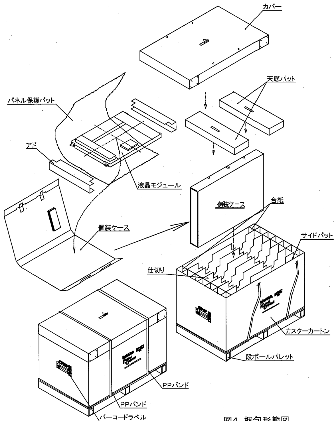
図4. 梱包形態図
