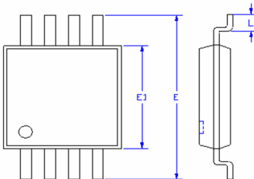
MSOP8
