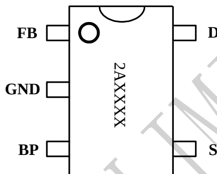
图 3 管脚封装图
