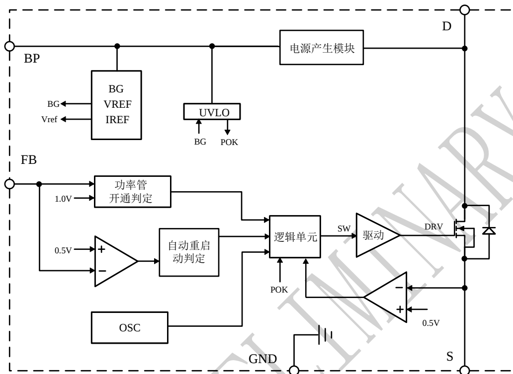
图 4 LP2701A 内部框图
