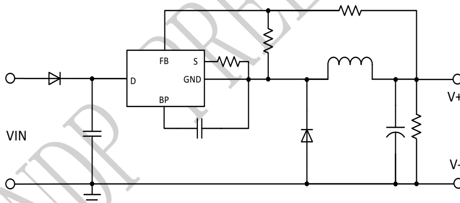
图 1 LP2701A 典型应用图
