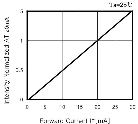
Fig. 2 I_v - I_F
