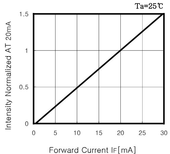
Fig. 2 I_v - I_F
