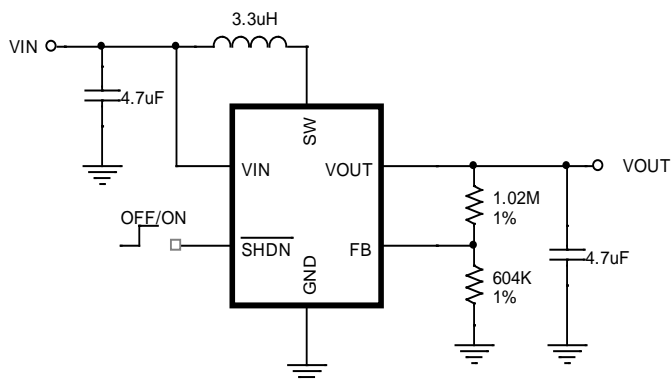
Figure1.Vout=3.3V
