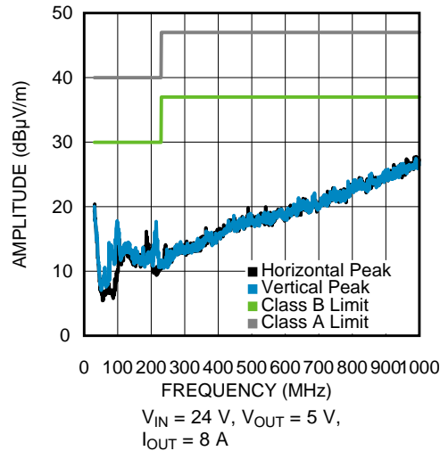
Figure 52. Radiated EMI (EN 55022)
