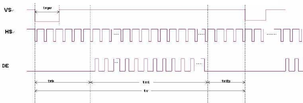
场时序图
