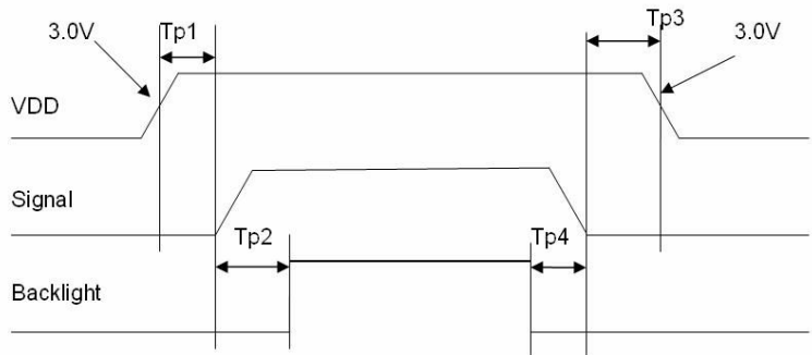
模块电源开/关时序
