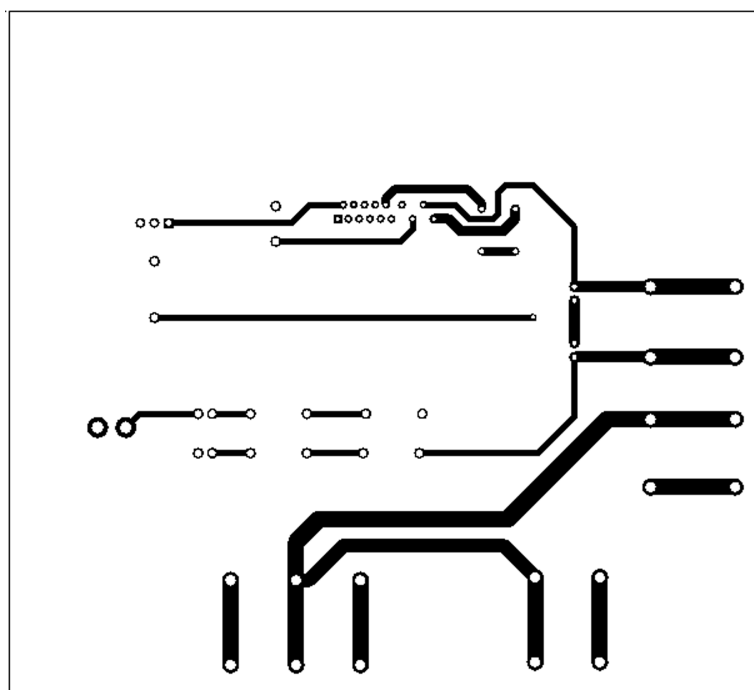
Top Layer
