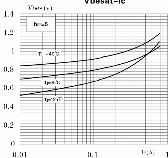
V_{besat} - I_c
