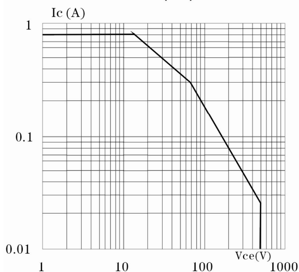
SOA(DC)
