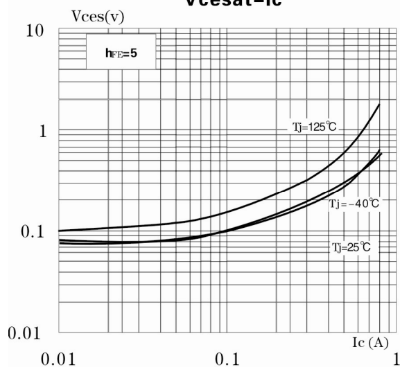
V_{cesat} - I_c
