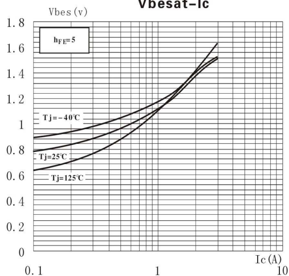
V_{besat}-I_c
