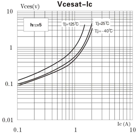
V_{cesat} - I_c
