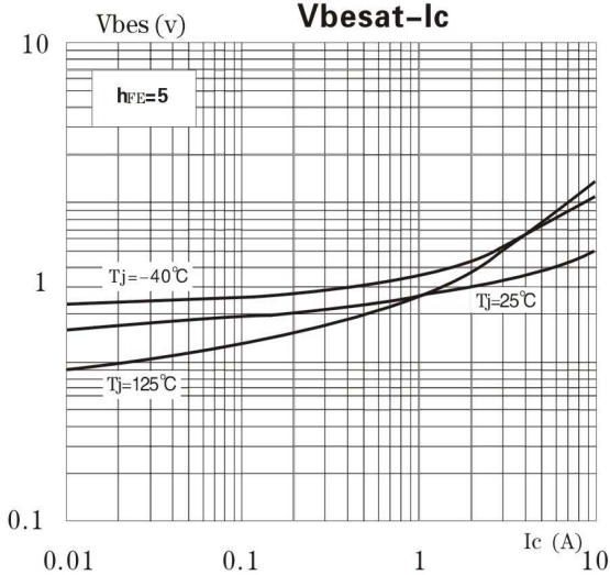
V_{besat} - I_c
