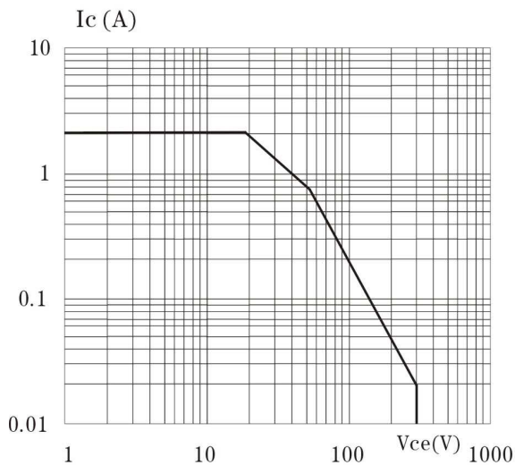
SOA(DC)
