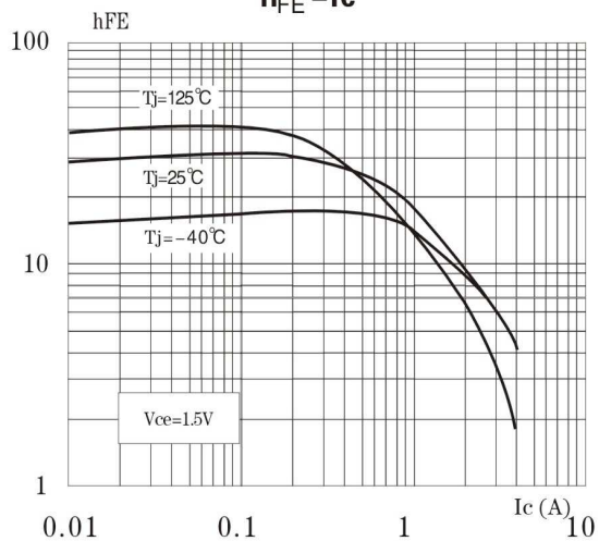
h_{FE} - I_c
