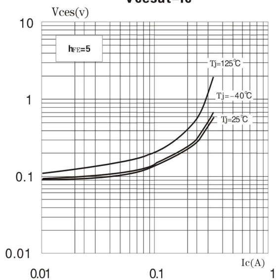
V_{cesat} - I_c
