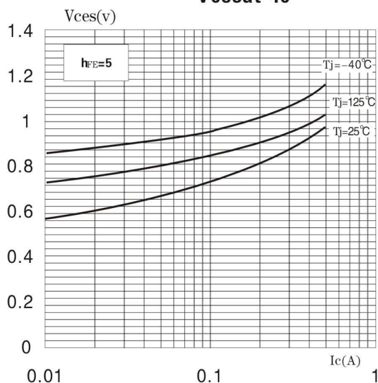
V_{cesat} - I_c
