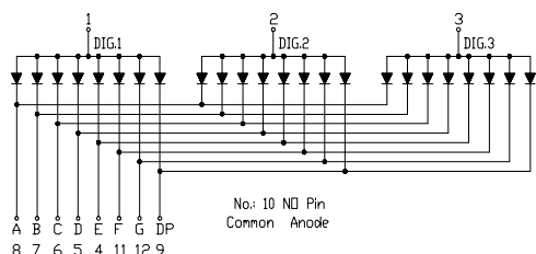
LD3031B (Common Anode)
