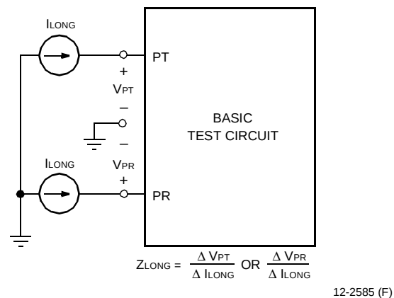
Figure 10. Longitudinal Impedance
