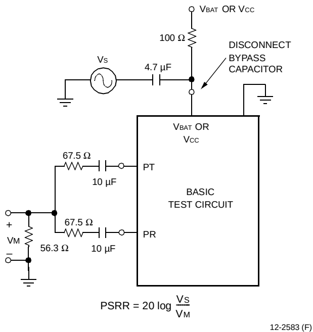
Figure 8. Longitudinal PSRR
