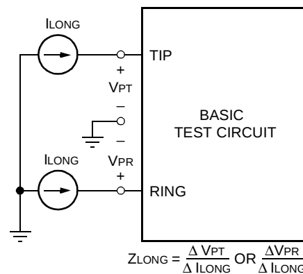
Figure 8. Longitudinal Impedance
