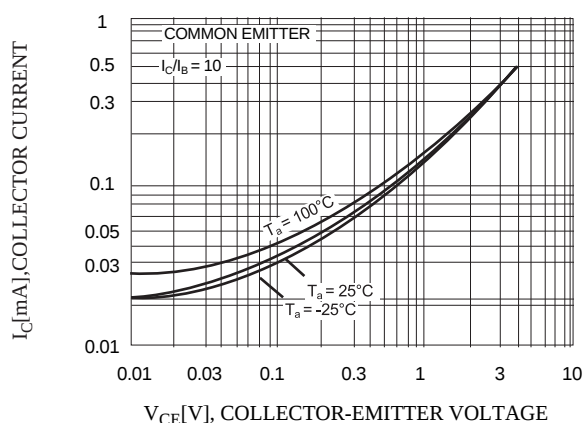
Fig.3 V_{CE(sat)} - I_C
