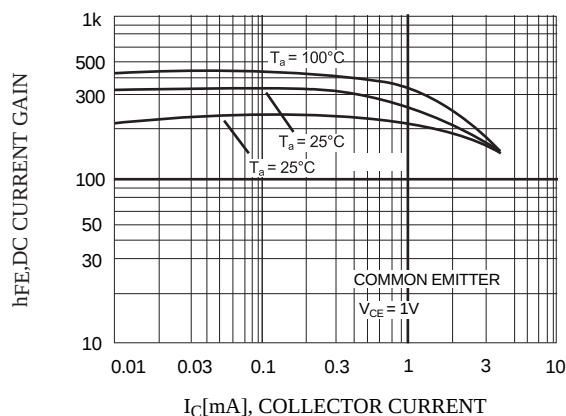
Fig.2 h_{FE} - I_C
