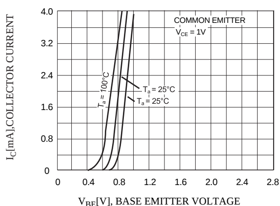
Fig.4 I_C - V_{BE}
