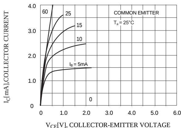
Fig.1 I_C - V_{CE}
