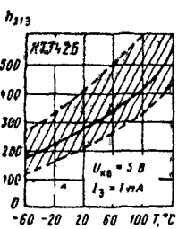
Зона возможных положений зависимости статического коэффициента передачи тока от температуры
