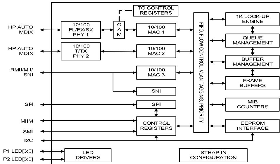
KSZ8893FQL
