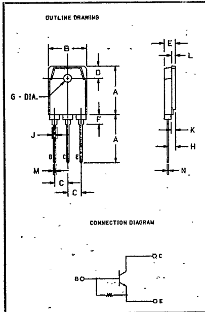
1000 Volt KS031KA0 Outline Drawing
