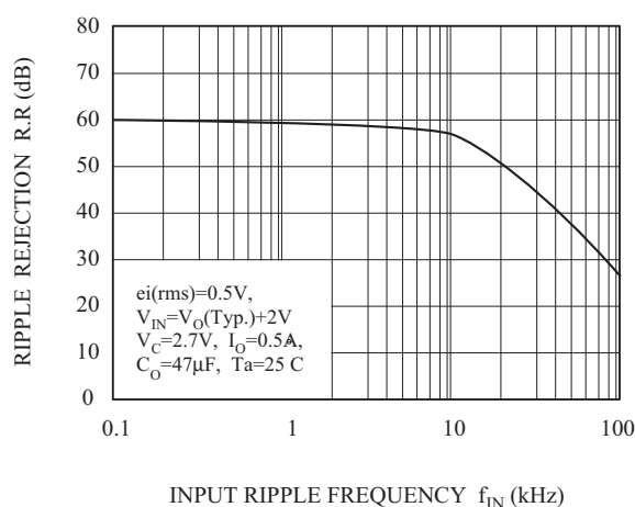
Fig. 13 f_{IN} - R.R
