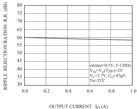
Fig. 14 I_{OUT} - R.R
