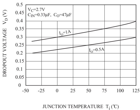
Fig. 11 T_J - V_D
