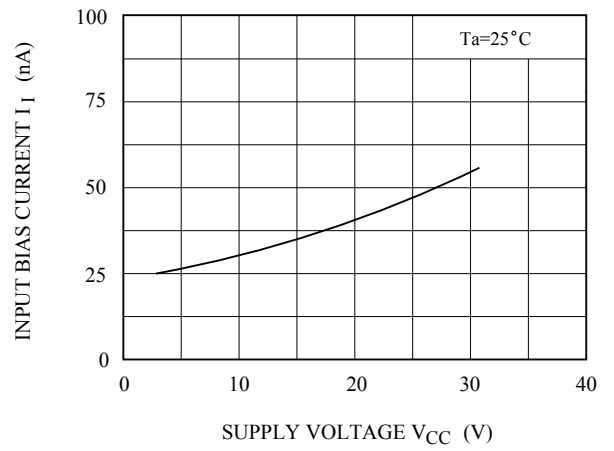
V_{CC} - I_I
