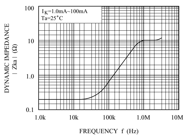
|Z_{ka}| - f
