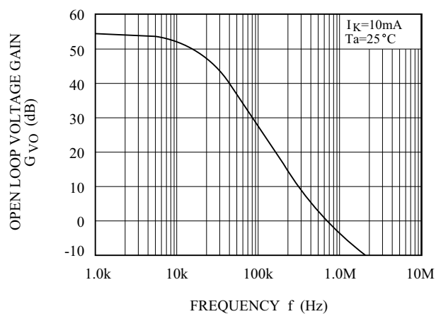
G_{VO} - f
