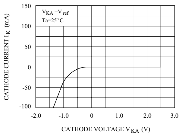
I_K - V_{KA}
