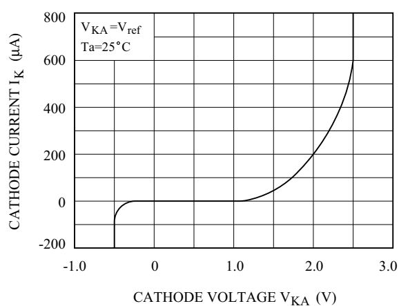
I_K - V_{KA}
