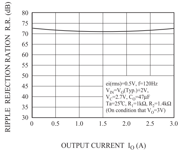
Fig. 11 V_{IN} - R·R
