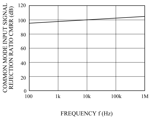
CMRR - f
