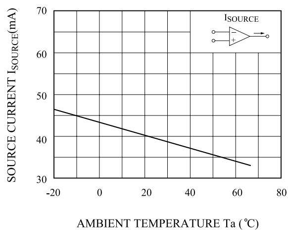
I_{SOURCE} - T_a
