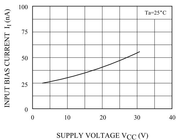
V_{CC} - I_I
