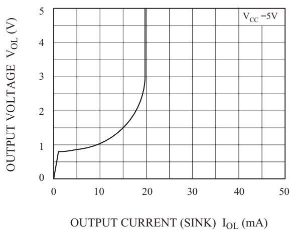
V_{OL} - I_{OL}
