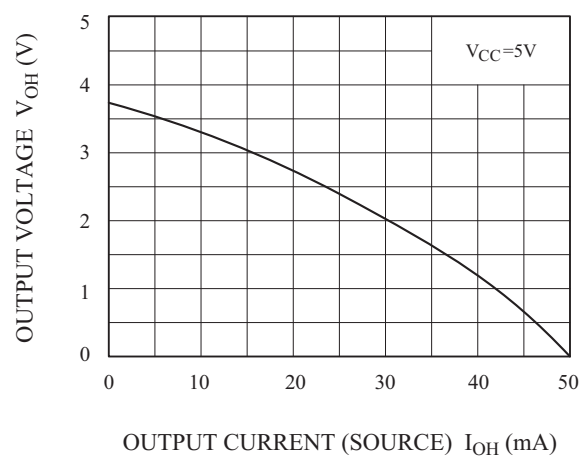
V_{OH} - I_{OH}
