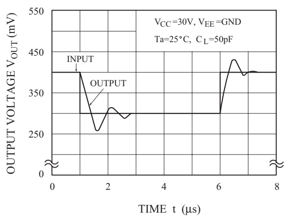
V_{OUT} - t
