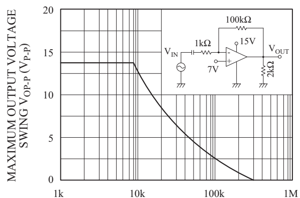
V_{OP-P} - f
