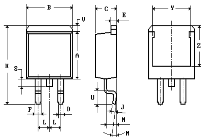
Корпус ТО-263
