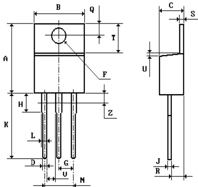
Корпус ТО-220 (КТ-28-2)
