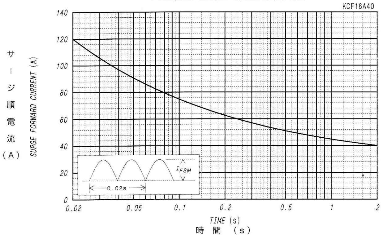
サージ順電流定格 SURGE CURRENT RATINGS
