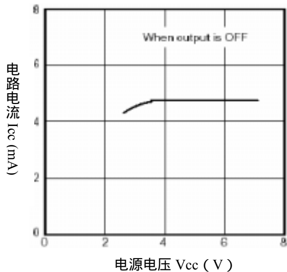
电路电流随电源电压的变化率
