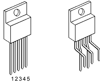
NJM2367TA2050
