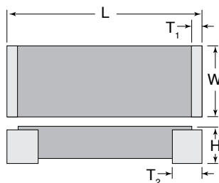
2512 size
