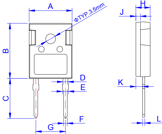
TO-247J-2L
