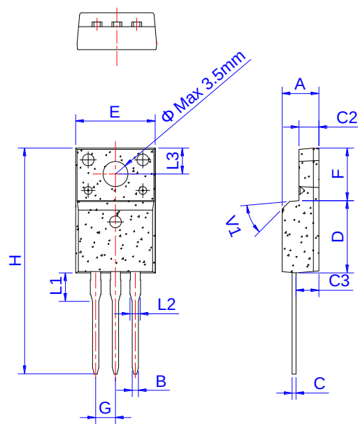
TO-220F Ins
