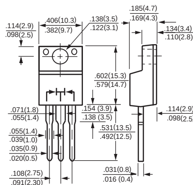
ITO-220
