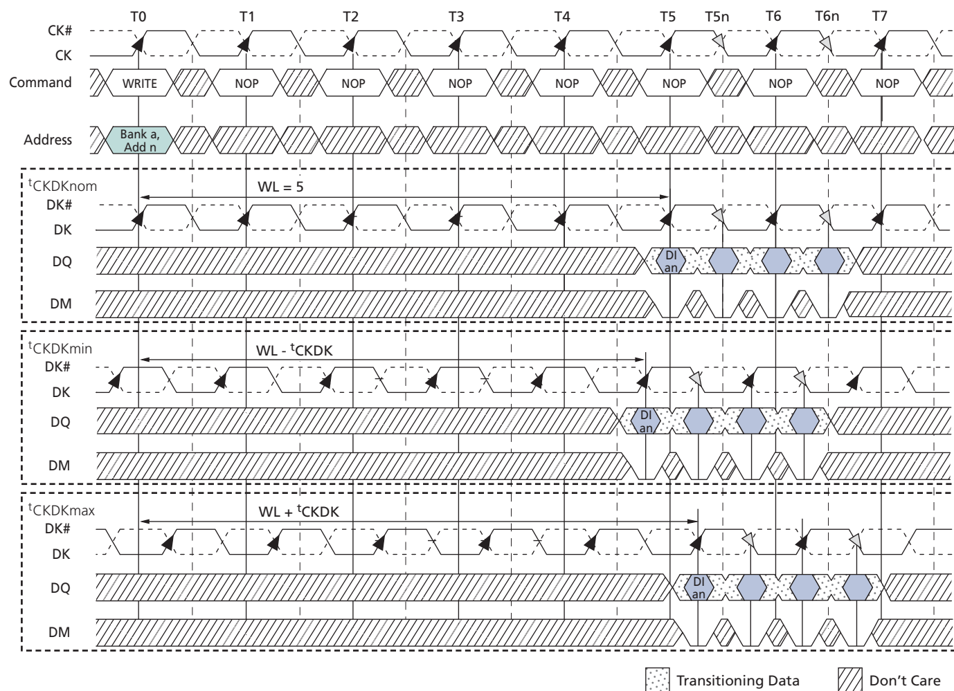
Figure43: WRITE Burst
