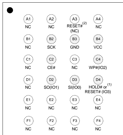
4x6 Ball Array
